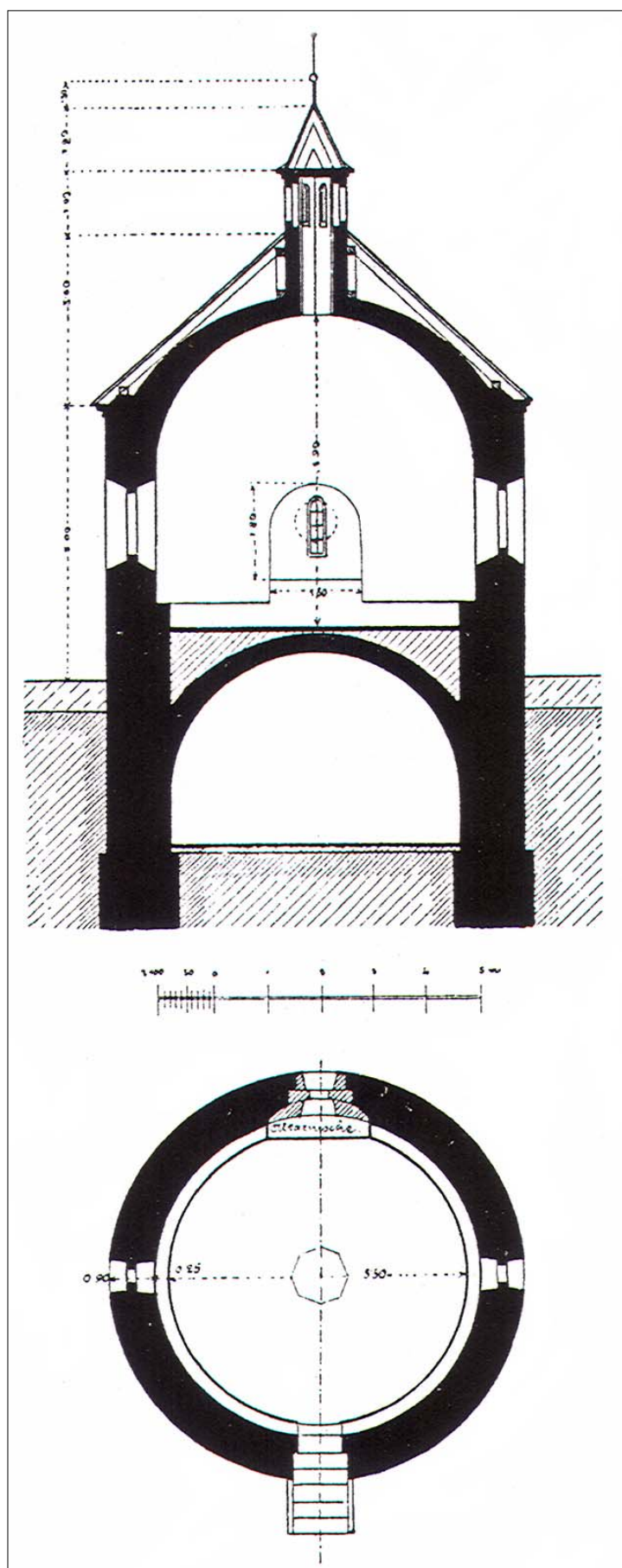
Karner. Zaměření půdorysu a řezu příčného podle A. Prokopa. Převzato z : A. Prokop, 1904, Bd. I, s. 121, obr. 151.
