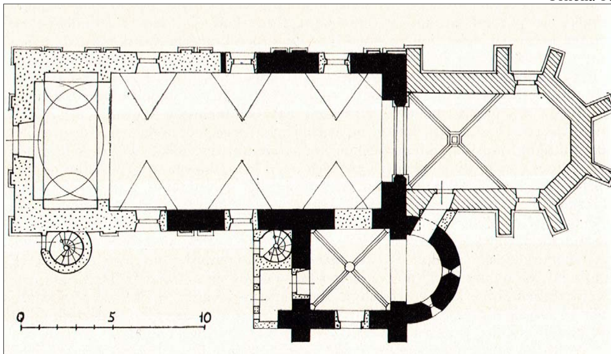
Trstěnice u Znojma, kostel Povýšení sv. Kříže. Půdorys se stavební analýzou podle K. Benešové (černě zdivo 13. stol., šrafovaně – gotika, tečkovaně – 16. až 19. stol.). Převzato z : K. Benešová, 1986, s. 305 – 312, zvl. s. 306.
