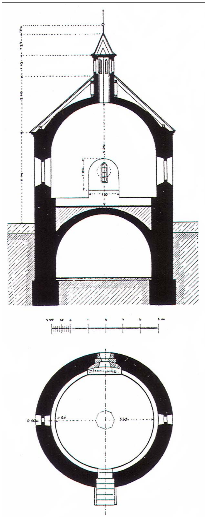
Karner. Zaměření půdorysu a řezu příčného podle A. Prokopa. Převzato z : A. Prokop, 1904, Bd. I, s. 121, obr. 151.
